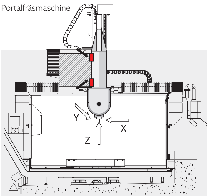
TRIMILL Portalfräsmaschine
